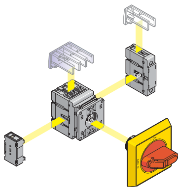
Установка на дверце
