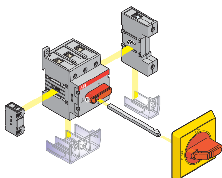
Установка на монтажной плате или на DIN-рейке
